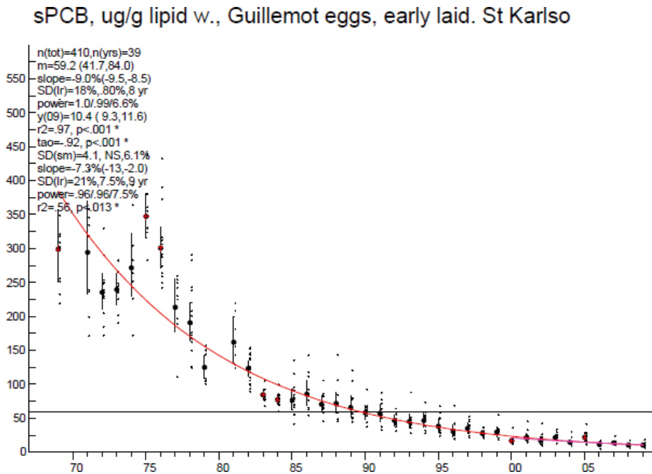
Figure 2.3.6.2-I: Example of time series of PCB concentrations in guillemot eggs from Stora Karlsö (Metaller och organiska miljögifter i marin biota, trend- och områdesövervakning. Sakrapport till nationella miljöövervakningen. Överenskommelse 2121011, dnr 235-3366-10Mm).
