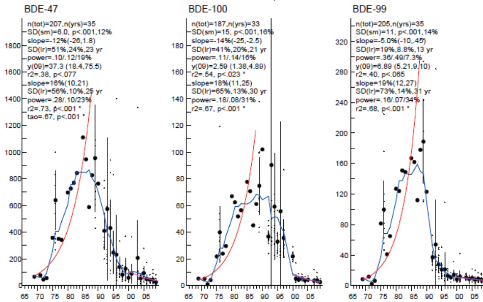
Figure 2.3.6.3-II: Example of a time series for BFRs at Stora Karlsö. (Metaller och organiska miljögifter i marin biota, trend- och områdesövervakning. Sakrapport till nationella miljöövervakningen. Överenskommelse 2121011, dnr 235-3366-04Mm).
