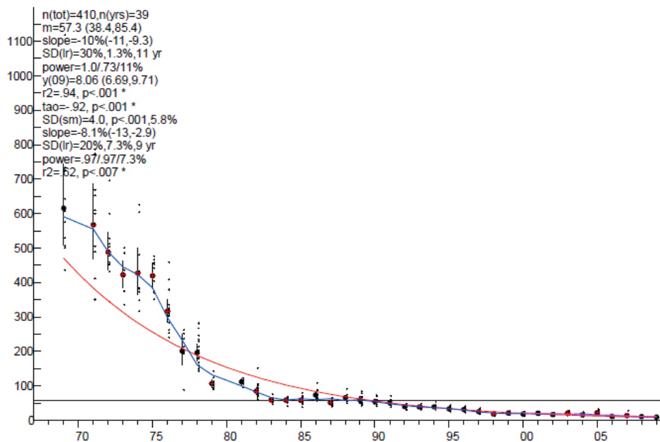
Figure 2.3.6.4-I: Example of a time series for sDDT at Stora Karlsö (sDDT = total DDT, the sum of the concentrations of DDT and its metabolites DDE and DDD). (Metaller och organiska miljögifter i marin biota, trend- och områdesövervakning. Sakrapport till nationella miljöövervakningen. Överenskommelse 2121011, dnr 235-3366-10Mm).
