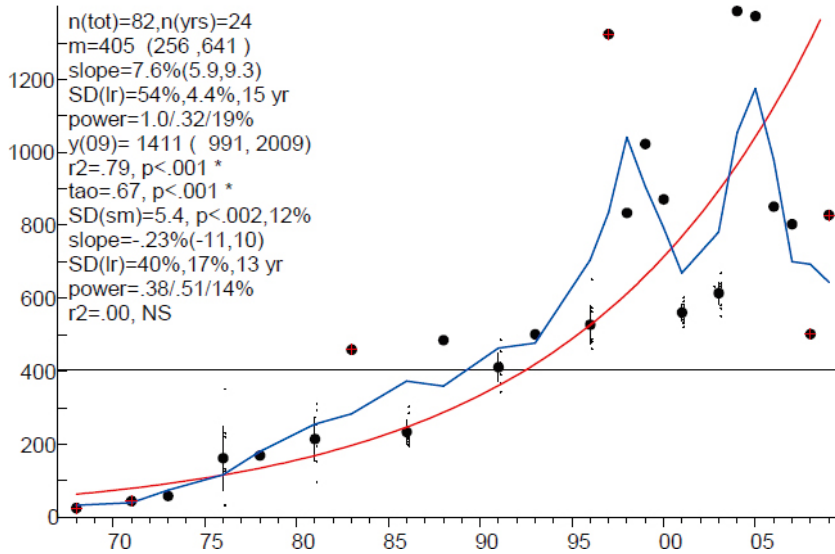
Figure 2.3.6.5-I: Example of a time series for PFOS at Stora Karlsö (Metaller och organiska miljögifter i marin biota, trend- och områdesövervakning. Sakrapport till nationella miljöövervakningen. Överenskommelse 2121011, dnr 235-3366-10Mm).
